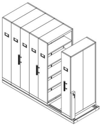
CPT-6 2540(L) x 914(W) x 1980(H) mm.
