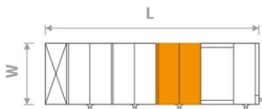
CPT-6 + CPT-E2 (CPT-8)
