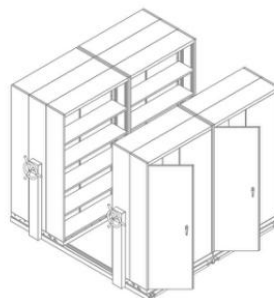
CPT-205 (2 แถว) 2540(L) x 2440(W) x 2250(H) mm.
