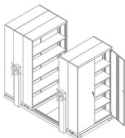
CPT-105T 2540(L) x 1000(W) x 2250(H) mm.
