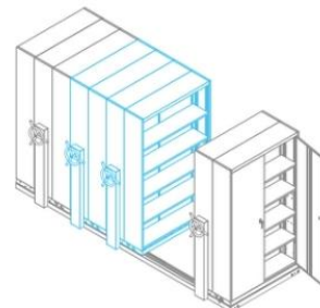
CPT-109T 3820(L) x 1000(W) x 2250(H) mm.
