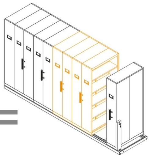
CPT-10 3820(L) x 914(W) x 1980(H) mm.
